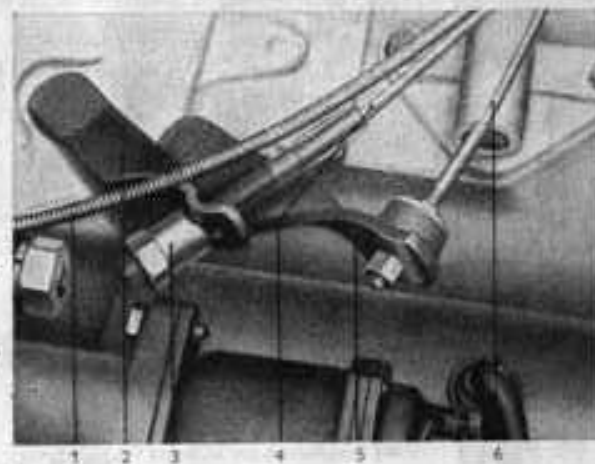
Bild 20 Einstellnippel am Kupplungsausrückhebel
