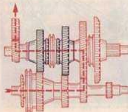
Bild 22. Kraftverlauf für den 2. Gang
