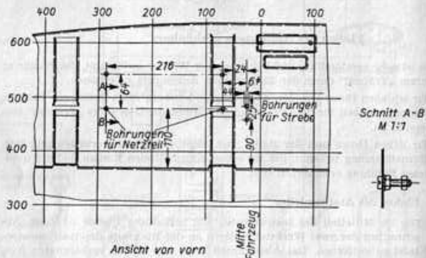
Bild 2. Skizze zum Bohren der Löcher für Befestigung des Netzteiltes und der Strebe
