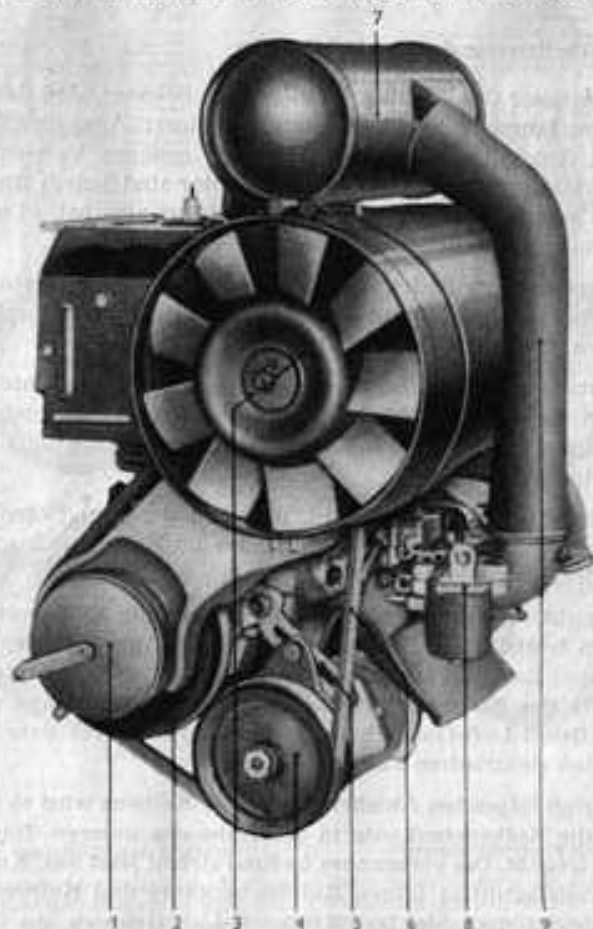
Bild 4. Motor, Seitenansicht
