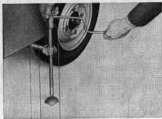
Bild 33. Wagenheber in Wagenheberstütze eingeführt
