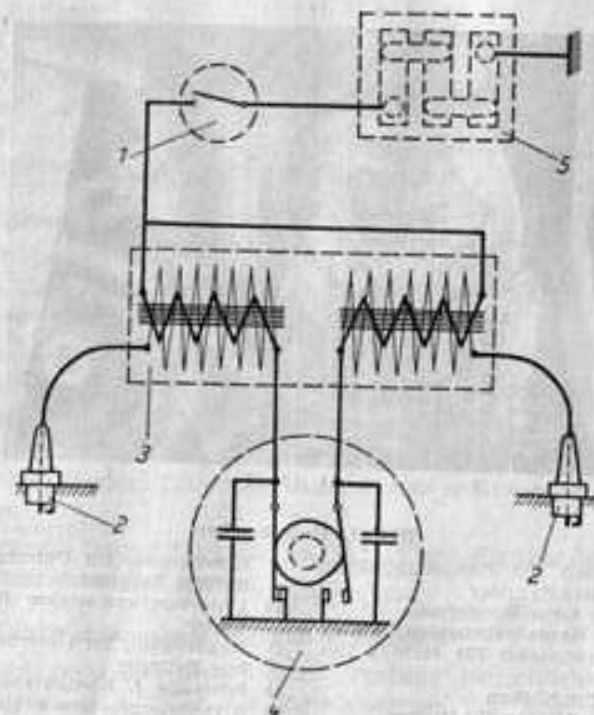
Bild 16. Schemadarstellung der Zündanlage
