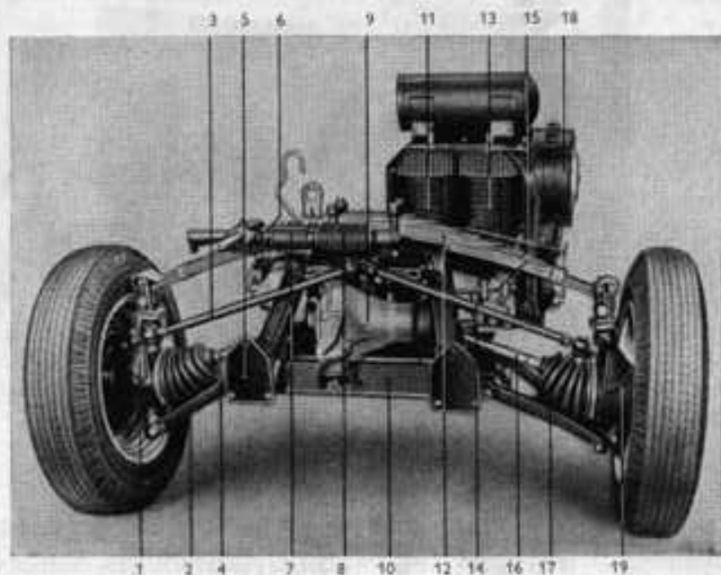
Bild 28. Triebwerkblock, auf Hilfsrahmen montiert (Ansicht von hinten)
