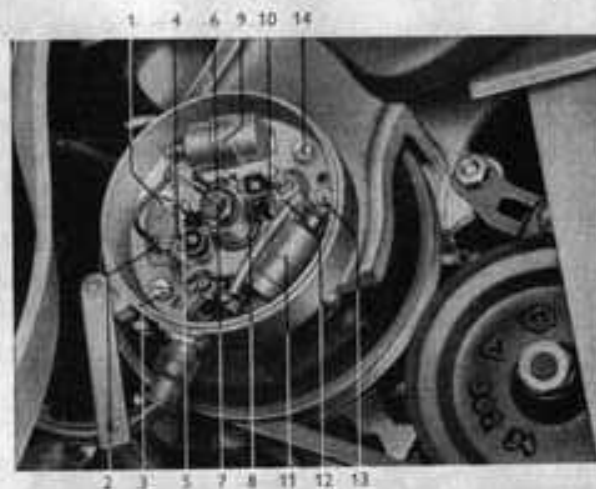
Bild 17. Unterbrecher
