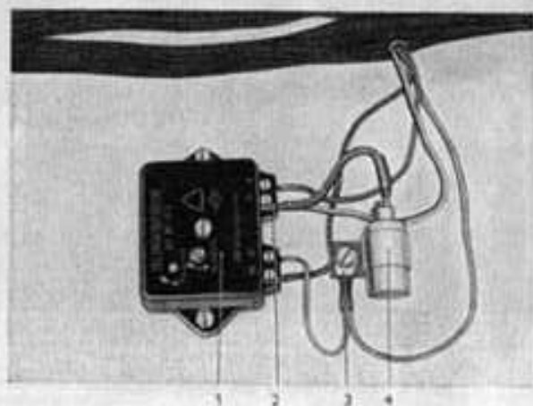
Bild 8. Abschirmung des Blinkgebers
