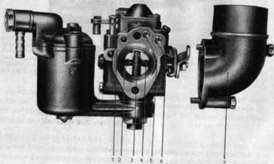
Bild 14. Vergaseransicht
