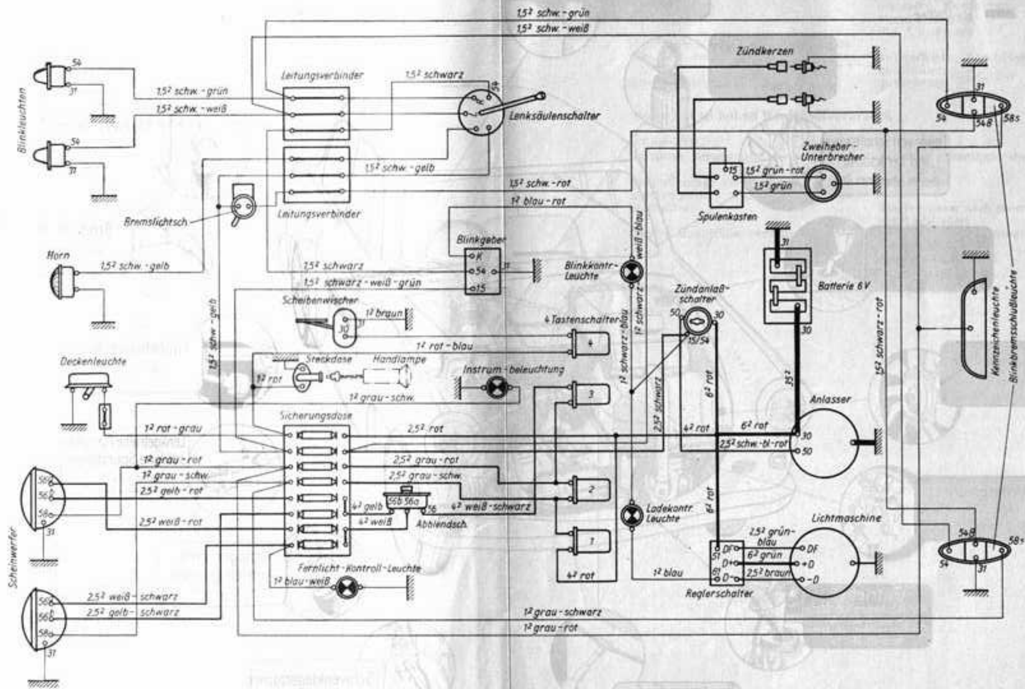
Bild 38. Schaltplan
