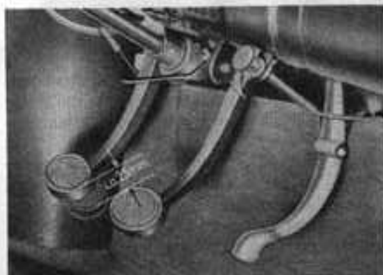
Bild 19 Kupplungspedalspiel
