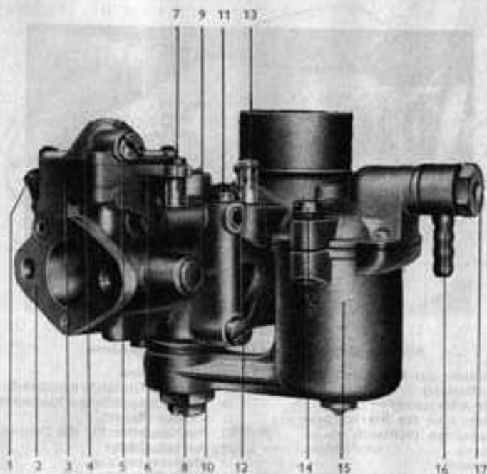
Bild 12. Vergaseransicht
