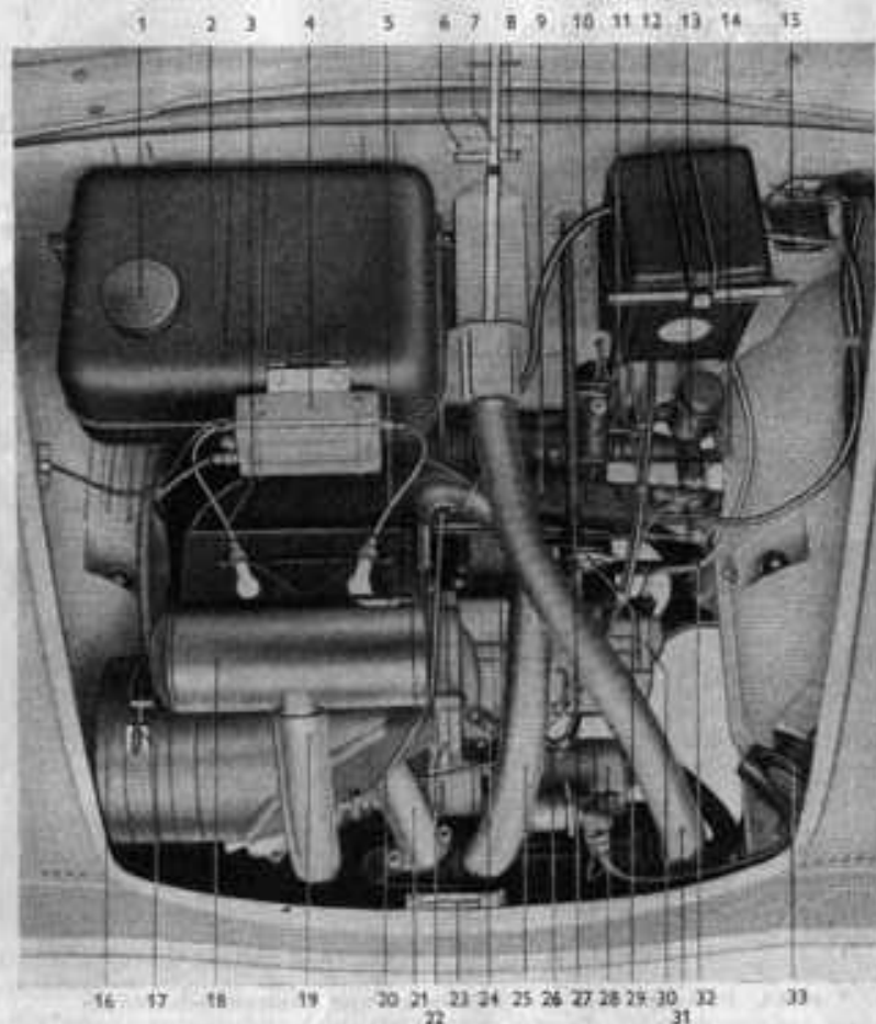
Bild 3. Blick unter die Motorhaube
