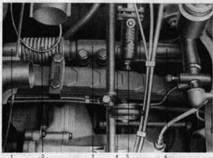
Bild 21. Lenkgetriebe
