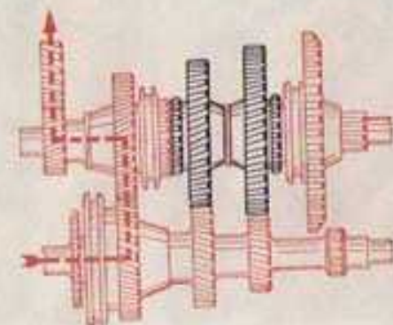
Bild 24. Kraftverlauf für den 4. Gang
