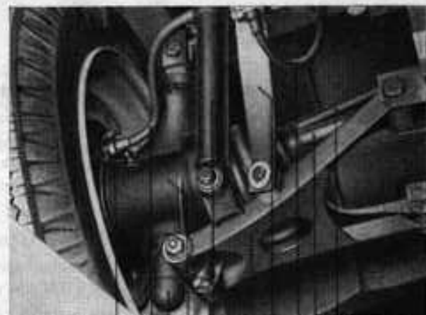
Bild 29. Vorderradaufhängung
