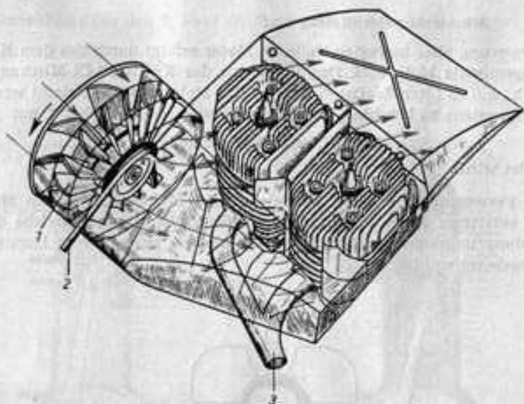
Bild 10 Schemadarstellung der Luftkühlung
