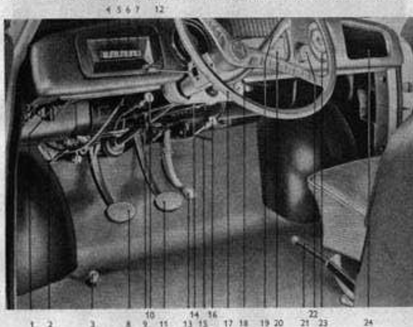
Bild 2. Übersicht über die Bedienungs- und Kontrolleinrichtungen
