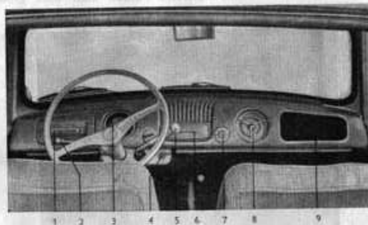
Bild 36. Instrumententafel
