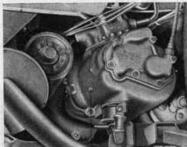
Bild 26. Getriebeöl-Kontrollschraube 1 Kontrollschraube
