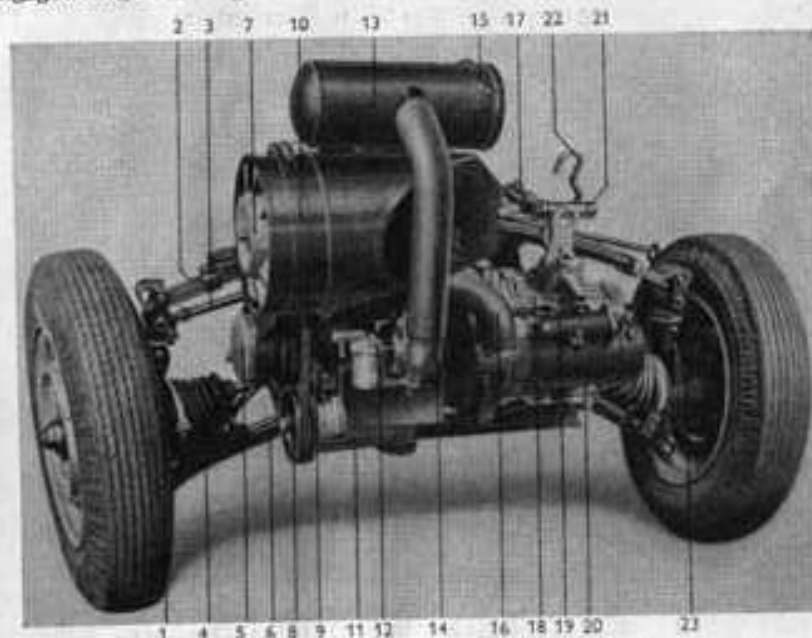
Bild 27. Triebwerkblock, auf Hilfsrahmen montiert (Ansicht von vorn)
