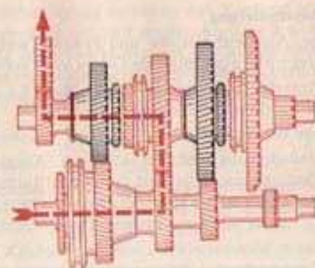
Bild 23. Kraftverlauf für den 3. Gang
