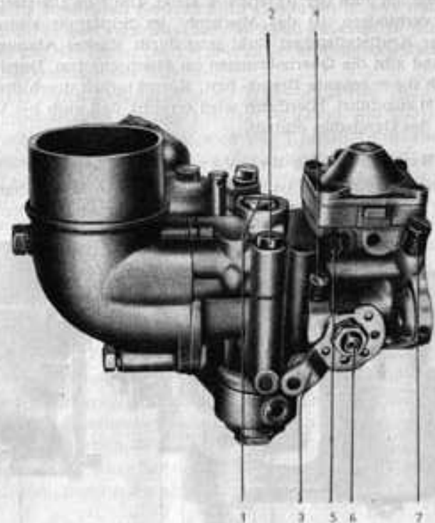
Bild 13. Vergaseransicht
