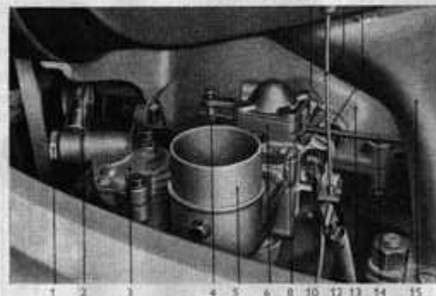
Bild 11. Vergaseranordnung am Kurbelgehäuse
