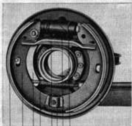
Bild 22. Bremsdeckplatte mit Radbremszylinder (Hinterrad)
