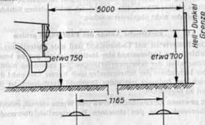
Bild 44 Maße für Scheinwerfereinstellung
