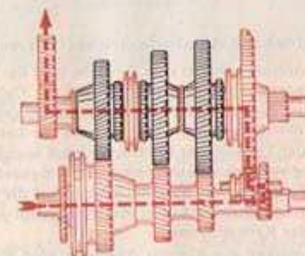
Bild 25. Kraftverlauf für den Rückwärtsgang
