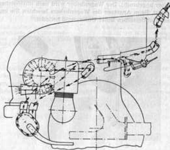
Bild 52 Warm- oder Kaltluftstrom geteilt zur Frontscheibe und in den Fahrgastraum
