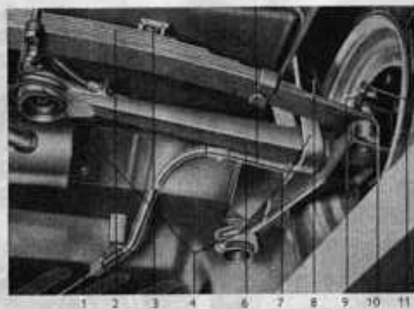
Bild 30. Hinterradaufhängung
