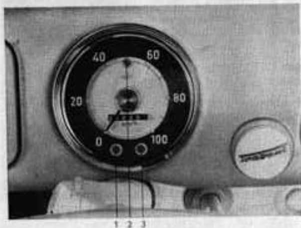
Bild 36a Kombinationsgerät (Tachometer)
