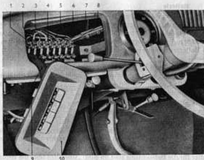
Bild 18. Zweckbestimmung der Sicherungen
