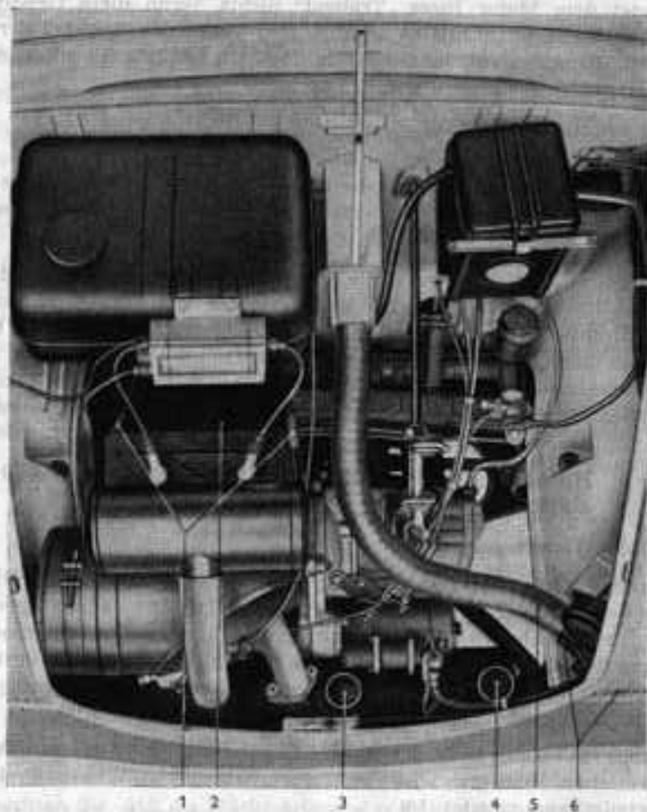
Bild 48. Frischluftführung für den Sommerbetrieb
