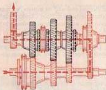
Bild 21. Kraftverlauf für den 1. Gang
