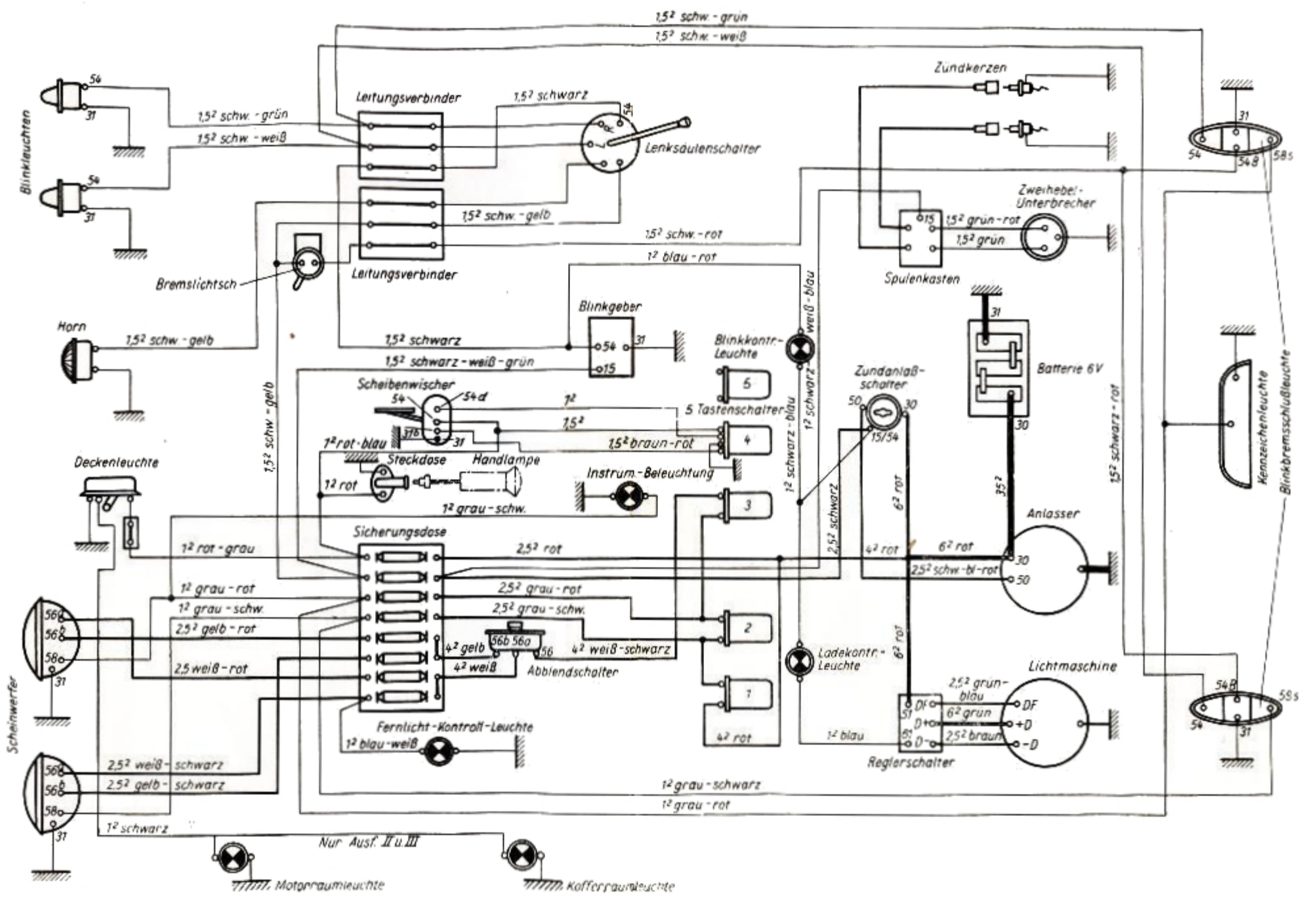
Schaltplan Trabant P50/P60 -1965
